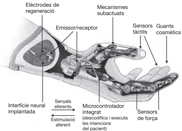
FIGURA 23. La mà bionica Cyberhand.
